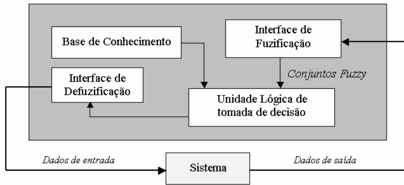
Figura 1: Diagrama de um controlador fuzzy (Fonte: Niittymäki,1998)
